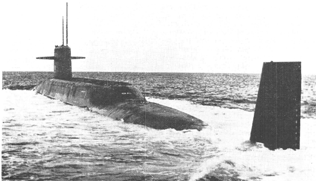
Polaris u-båd.
