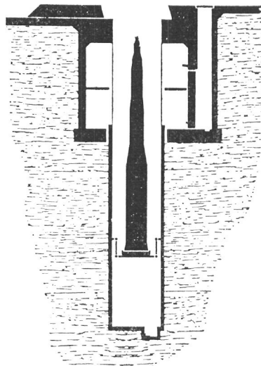
Skitse af underjordisk tilholdssted for raket med fast sprængstof (Minuteman).
